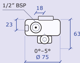
Stirnansicht
