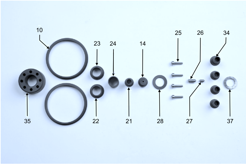
Abb.83: Verschleißteilsatz TSG
